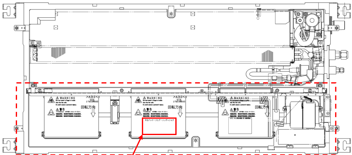
仕様銘板
