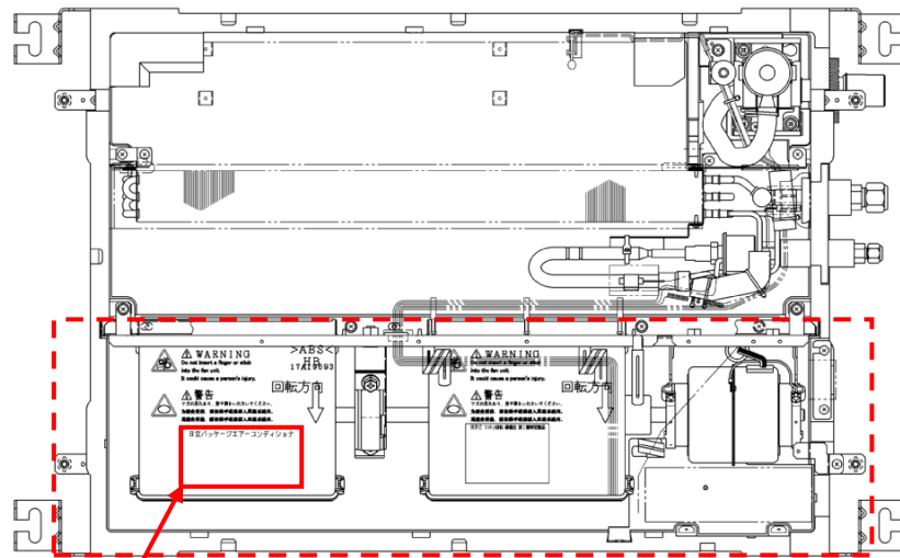
仕様銘板
